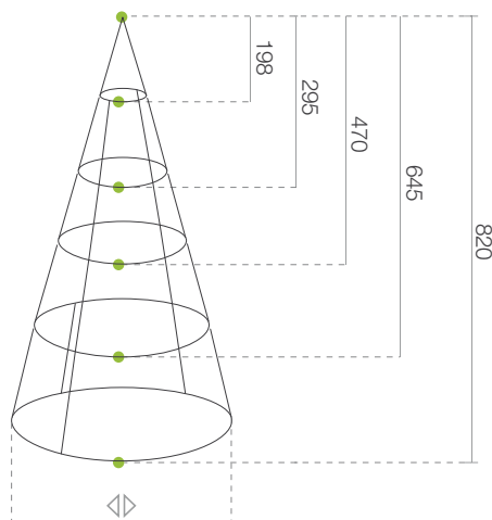
RZUT TECHNICZNY
