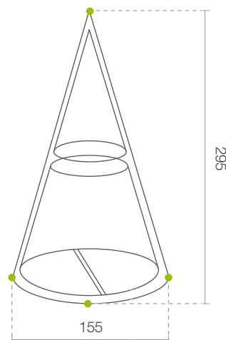
RZUT TECHNICZNY
